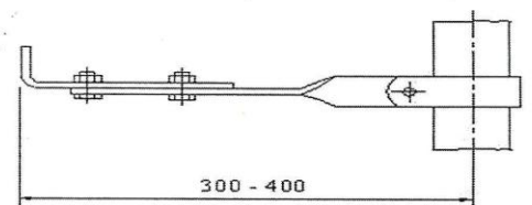
Кронштейн крепления (6)
