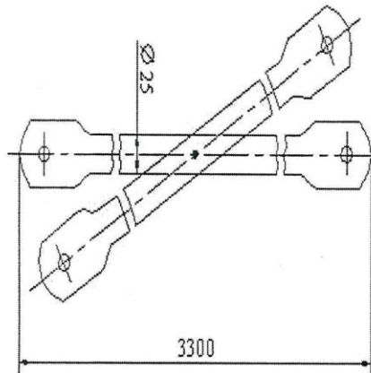
Диагональная связь (4)
