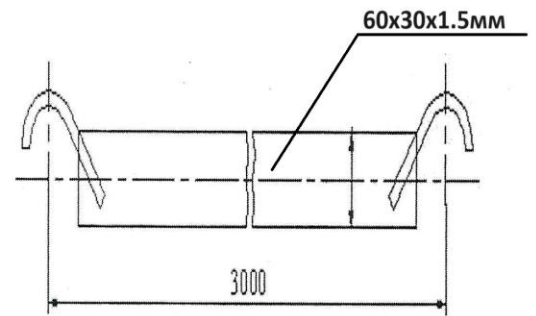
Ригель настила (7)
